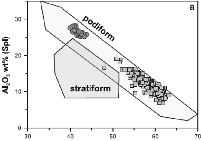
Şekil 10. Yüksek ve düşük Cr içerikli kromitlerin Al_2O_3 ve Cr_2O_3 içeriklerine göre karşılaştırılması ve sınıflanması (Uysal ve diğ., 2009'dan alınmıştır).
