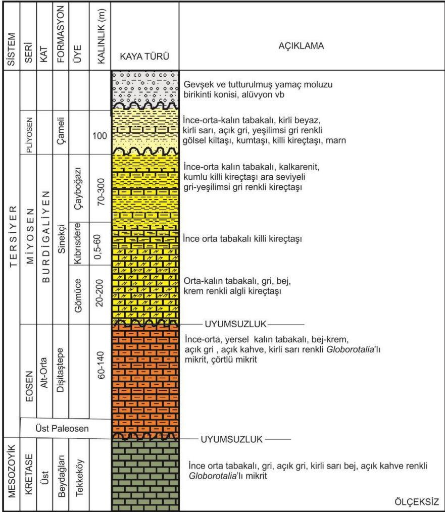
Şekil 13. Dalaman-Ortaca-Göcek ve çevresinin genelleştirilmiş stratigrafik dikme kesit (Darbaş ve Gül, 2017; Bilgin ve diğ. 1997’den değiştirilerek alınmıştır).
